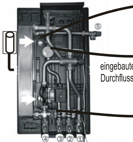
Warmwasserstation eingehängt
